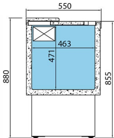
doorsnede EFB
