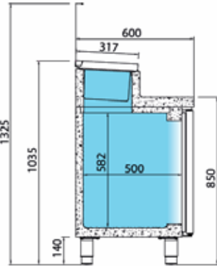
doorsnede BMPP
